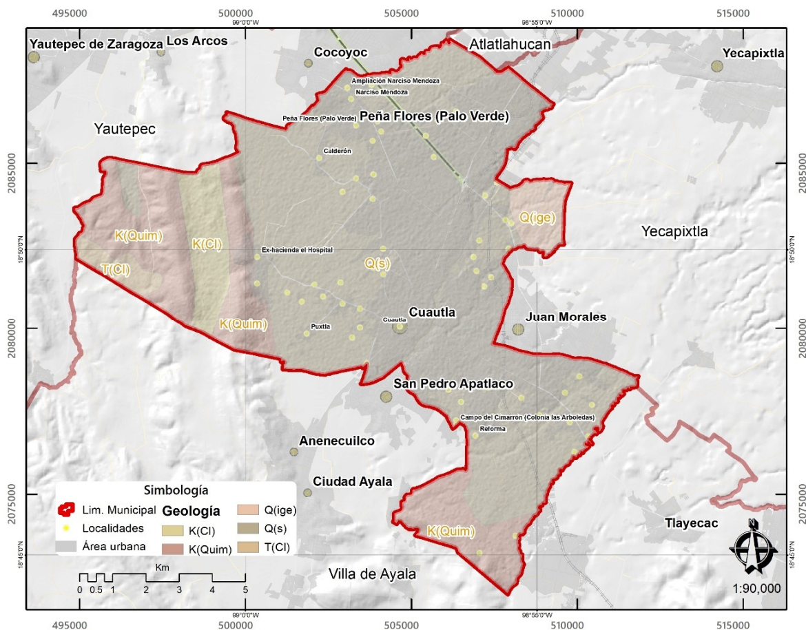
Tipos de roca presentes en el municipio
